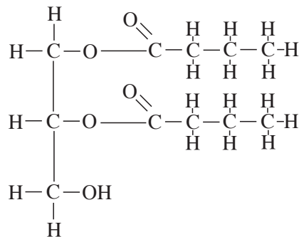
Fig. 15 A diglyceride.
