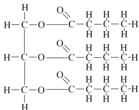
Fig. 16 A triglyceride.
