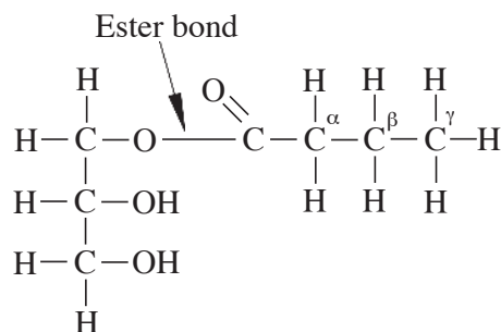
Fig. 14 A monoglyceride.
